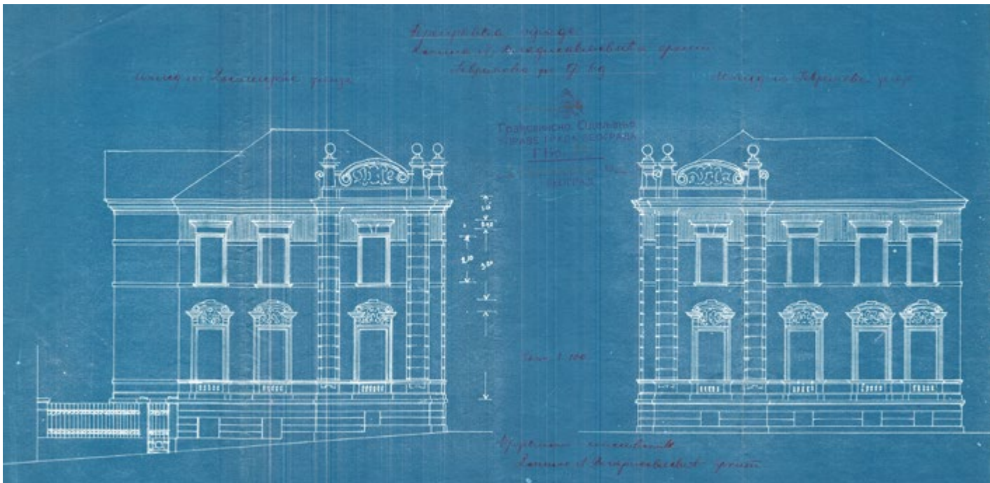
Сл. 2 / План уређивања зграде Данила Л. Владисављевића у Господар Јевремовој бр. 69, изглед фасада ка Јевремовој и Доситејевој улици, 1921. Извор: ИАБ, ОГБ, ТД ф 2-19-1921
