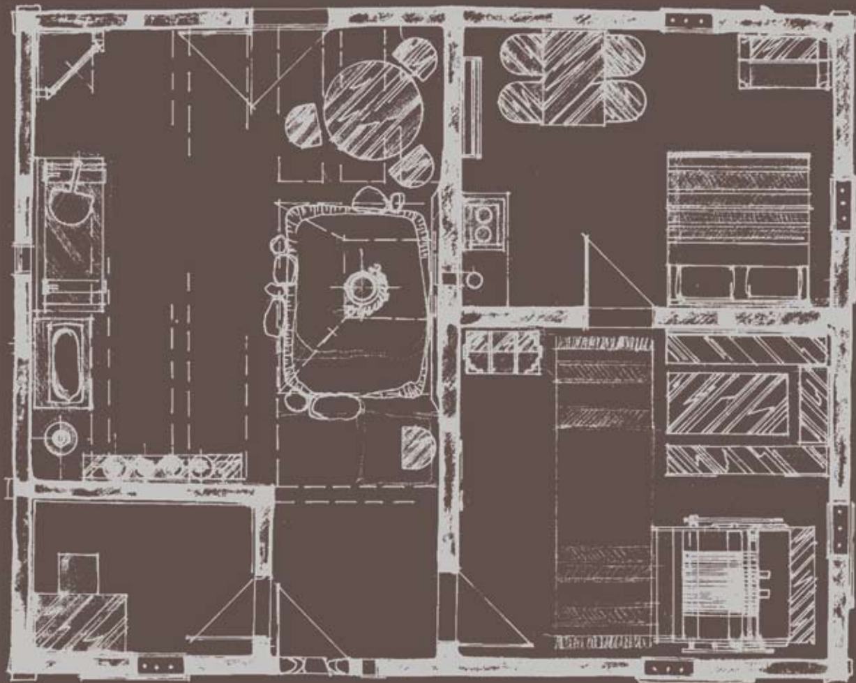
Кућа породице Матић у Вранићу, основа, цртеж Matić Family House in Vranić, ground plan, drawing
