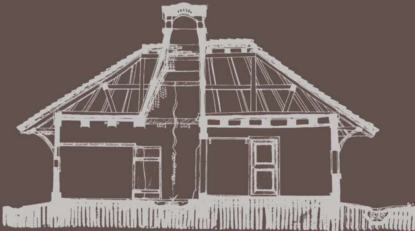
Кућа породице Матић у Вранићу, пресек, цртеж Matić Family House in Vranić, cross section, drawing
