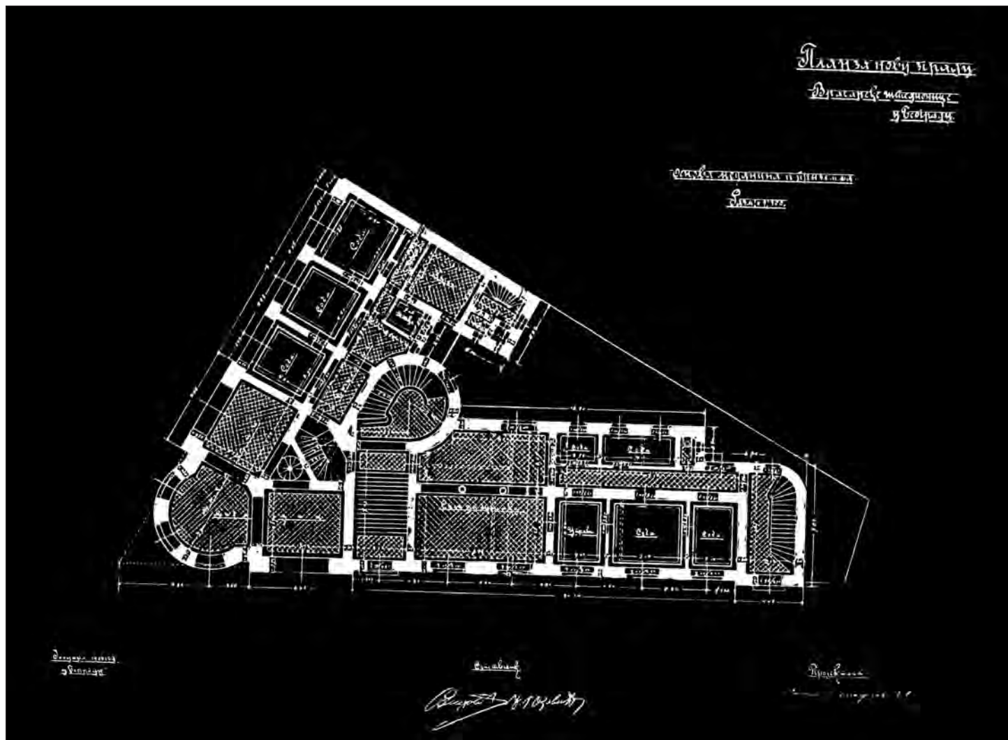
Сл. 1. Данило Владисављевић. Пројекат основе и приземља и мезанина Дома Врачарске штедионице, објављен у књизи »50 година рада инжењера Милоша Савчића 1889–1939«, Београд [1940]
