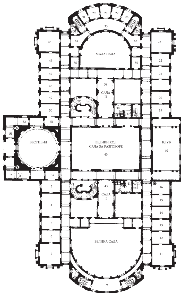
Сл. 4. Основа њриземља Скупштинске зграде
