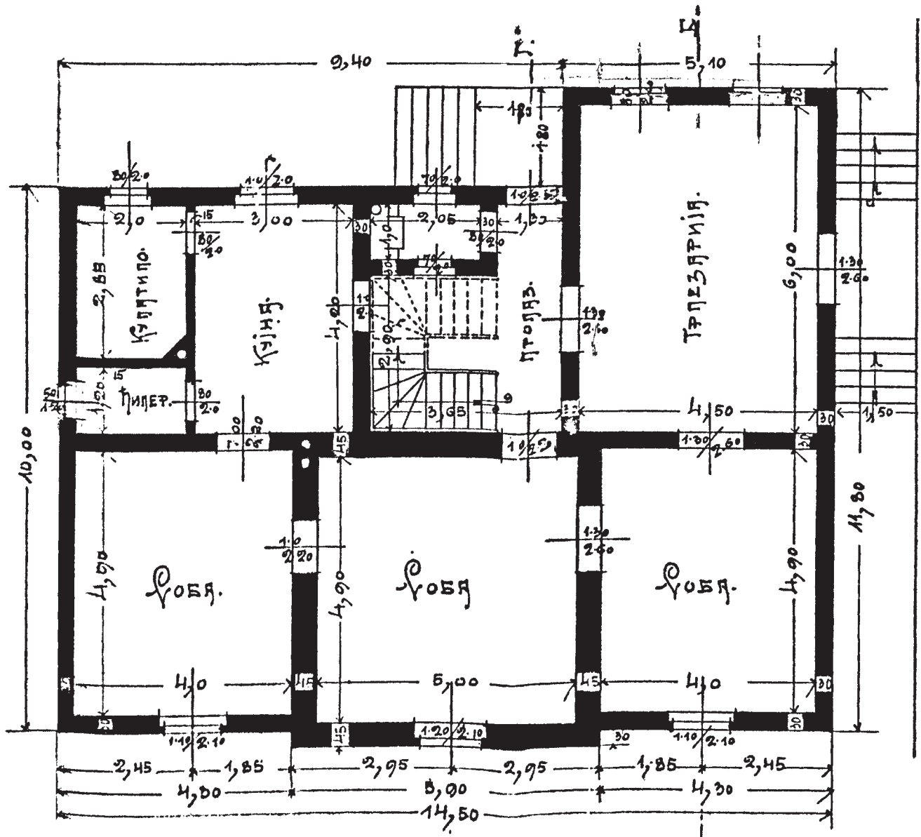
Сл. 1. Вила Боторић – основа приземља
