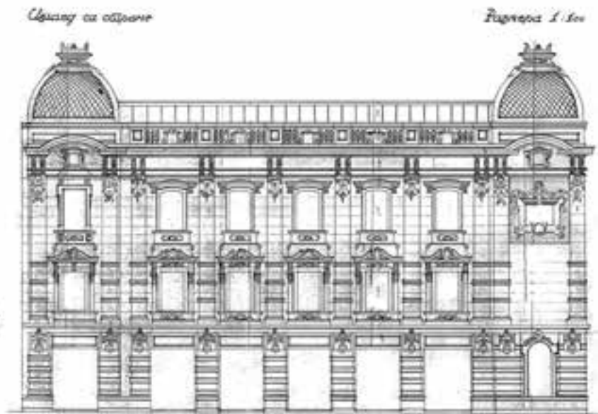
Сл. 5. Фасада крила у Херцејовачкој улици
