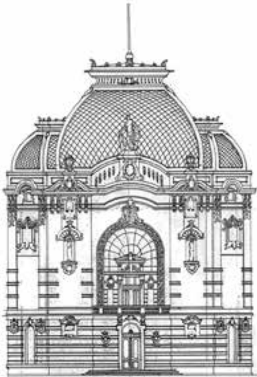
Сл. 4. Прочеље палате (планове на сл. 4–8 снимио инж. Драјомир Владимировић 1931. године, Документација завода за заштити споменика културе града Београда)
