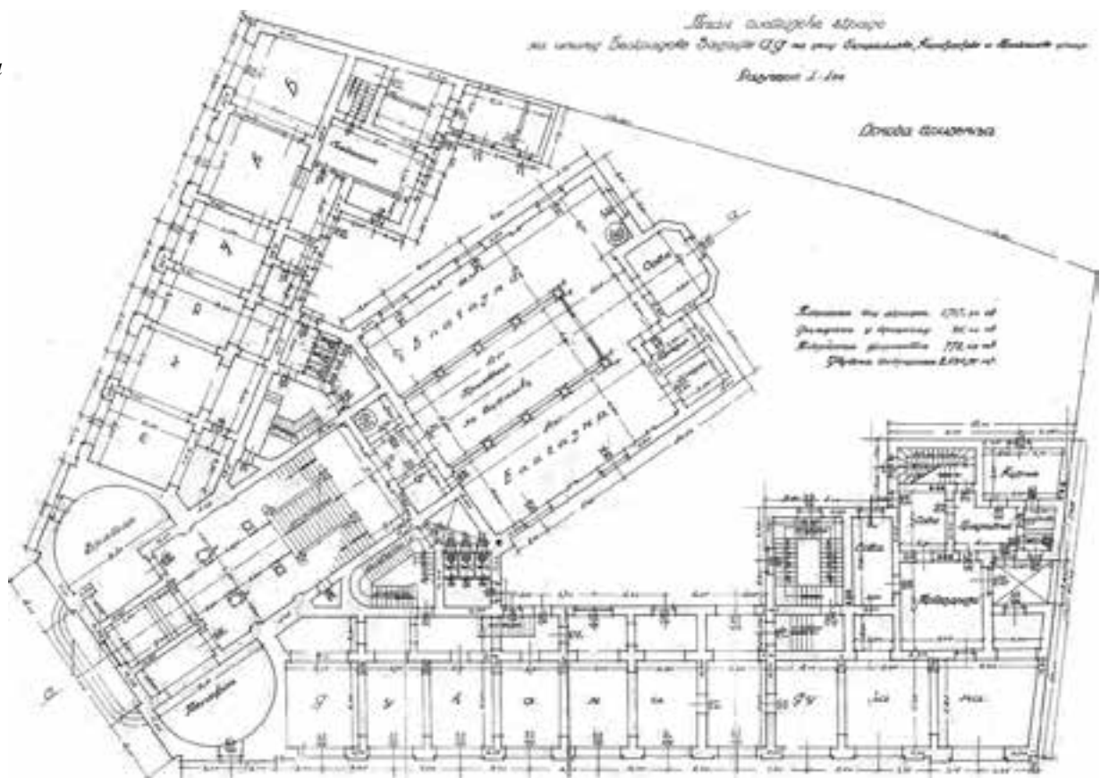
Сл. 6. Основа приземља
