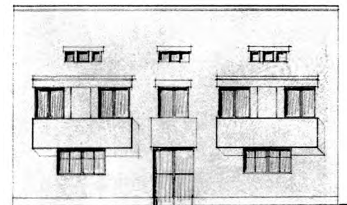
Сл. 1. Остали изглед сирајне куће Јована Карамате (према пројекту)
