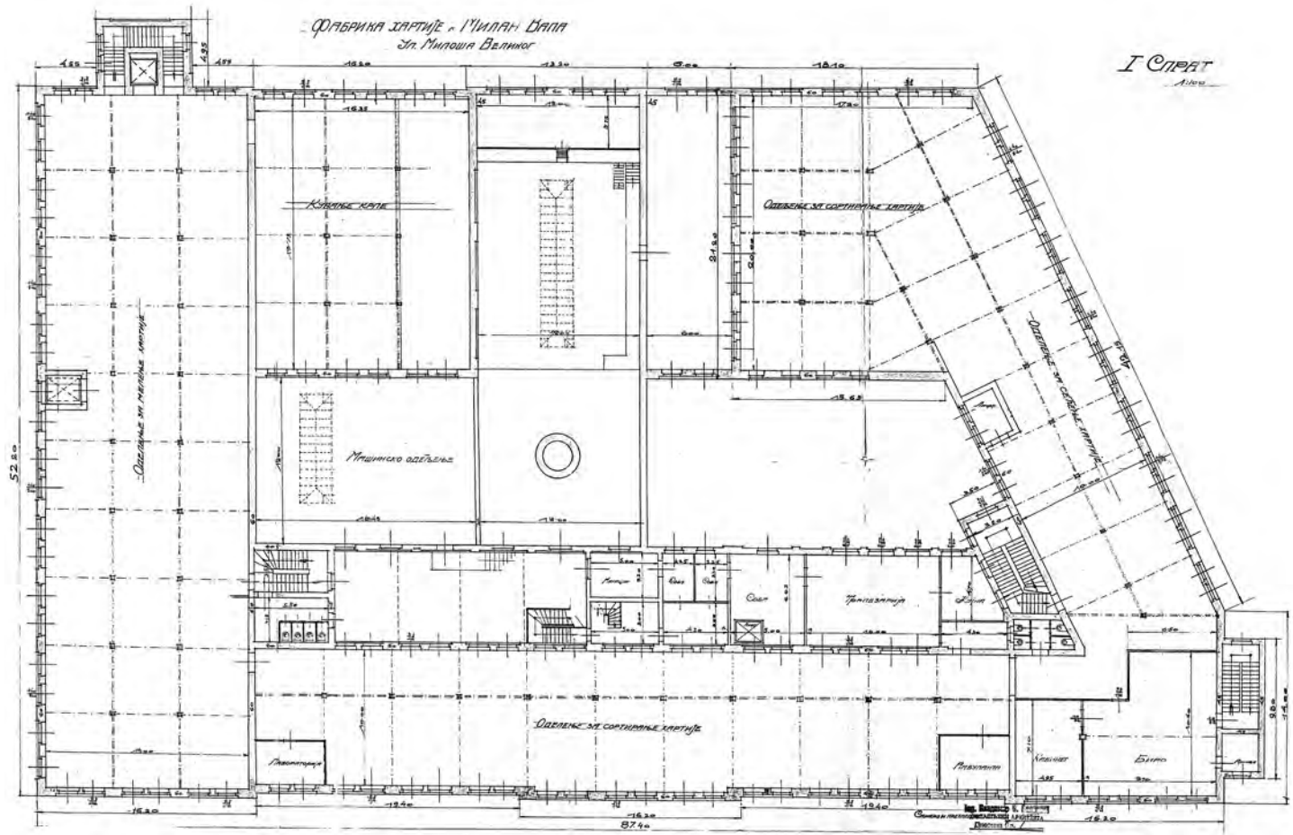
План фабрике хартије „Милана Вапа“ за Милоша Величког
