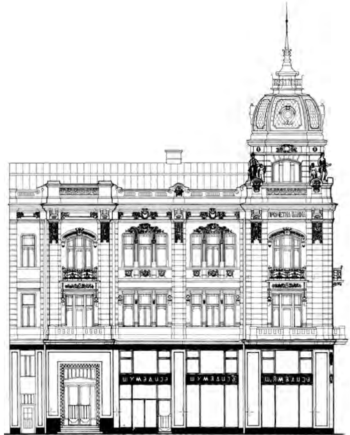
Сл. 2. Пројекат реконструкције фасаде, изглед из Змај Јовине улице. Израдили арх. Зоран Јаковљевић и арх. Слободан Појовић 1985. године (планови на сликама 2 и 3 чувају се у Документацији Завода за заштитију сјоменика културе града Београда)
