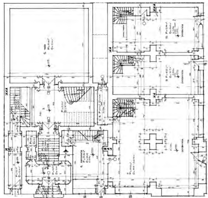
Сл. 3. Основа њриземља (снимио Ђорђе Мишировић, 1983)
