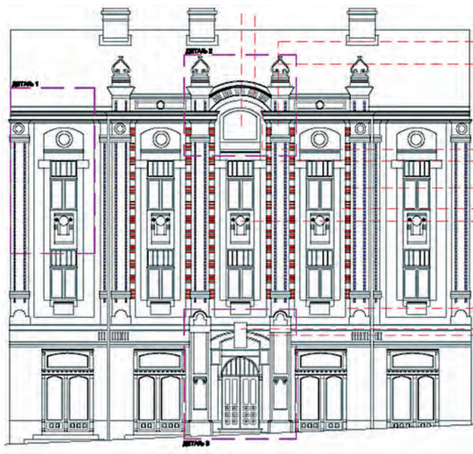
Сл. 10. Приказ фасаде зграде браће Николић, Њејшјева 11 (сцугенй: Бојана Живановић)
