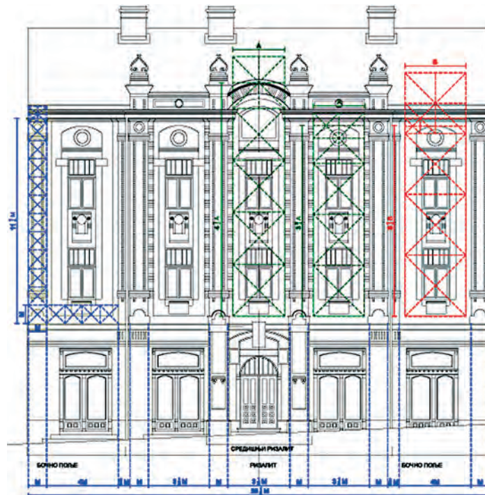
Сл. 11. Анализа фасаде зграде браће Николић, Њејшјева 11 (сцугенй: Бојана Живановић)
