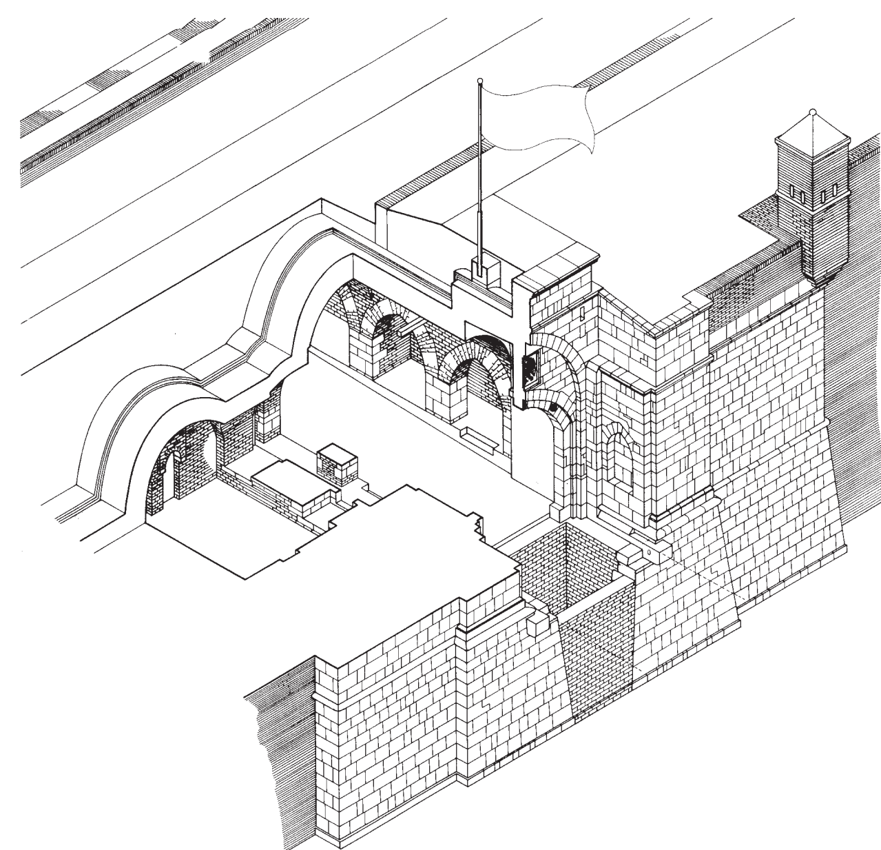
ИЗОМЕТРИЈСКИ ПРЕСЕК ISOMETRIC SECTION
