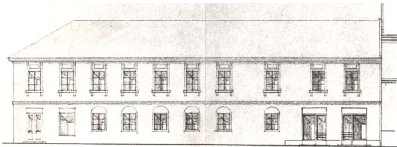
План главне фасаде, Главна улица Elevation facing, Glavna street
