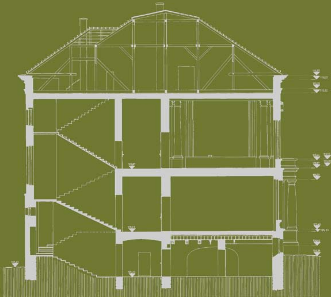
Палилука основна школа, попречни пресек Palilula Elementary School, cross section
