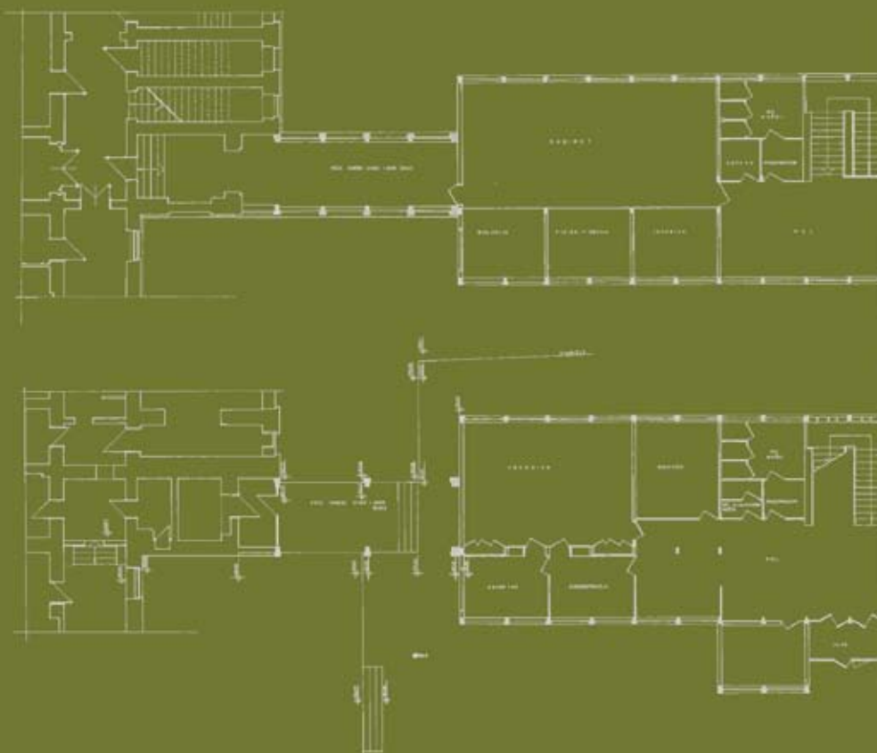
Палилулска основна школа - основа приземља и првог спрата Palilula Elementary School, ground floor and first floor plan
